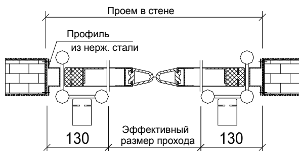
ВРТ4 двустворчатая (установка в несущую стену)
