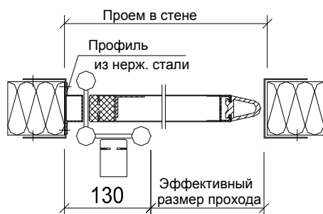
ВРТ4 одностворчатая (для стен из сэндвич-панелей)
