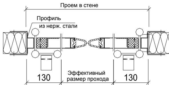
ВРТ4 двустворчатая (для стен из сэндвич-панелей)
