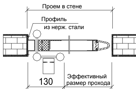
ВРТ4 одностворчатая (установка в несущую стену)
